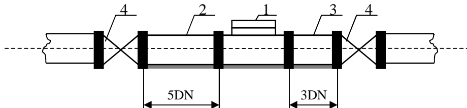
Рис. 3 Рекомендована схема встановлення лічильника води
